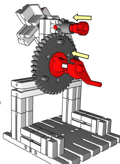
7. Wellenlager für Zahnräder
