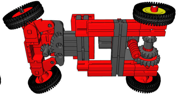
Durch Verschieben des Motors lassen sich 3 Geschwindigkeiten einstellen
