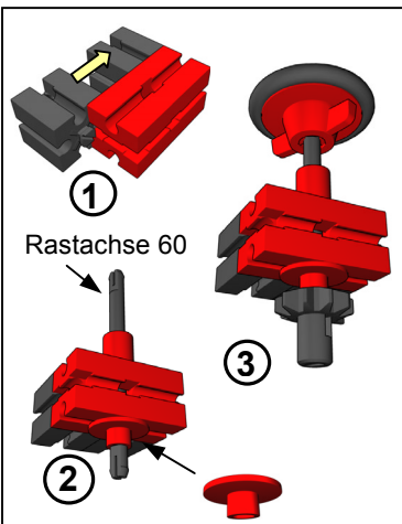
mit Achsschenkelenkung
