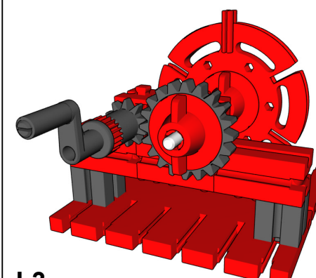
Antriebskurbel und Zähscheibe
