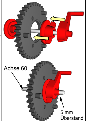
9. Zahnrad mit Kurbel
