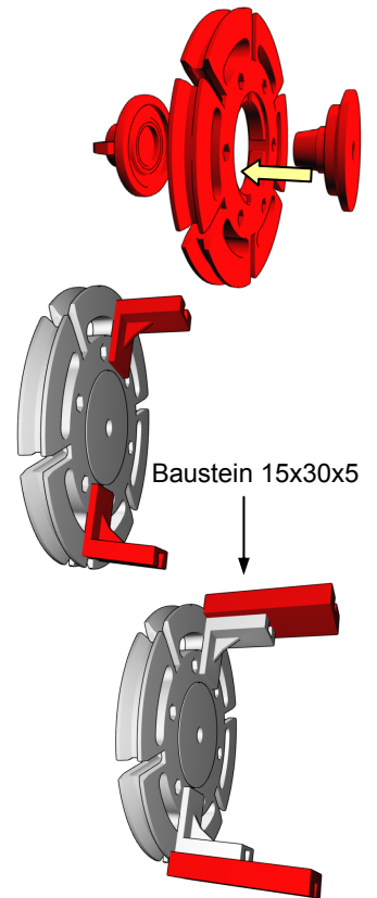
9. Zahnrad mit Kurbel
