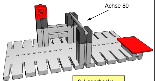
6. Lagerböcke
