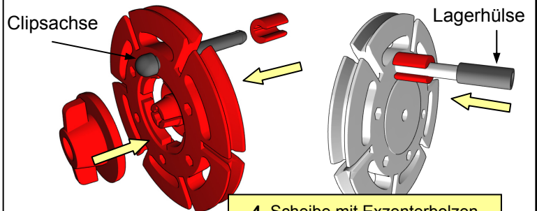
4. Scheibe mit Exzenterbolzen
