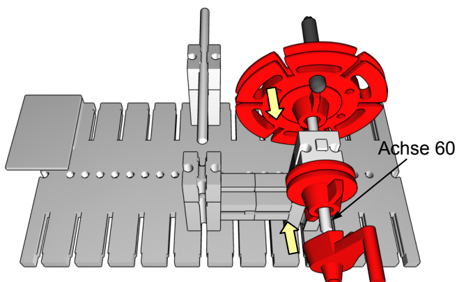
7. Einbau der Exzenter Scheibe mit Kurbel
