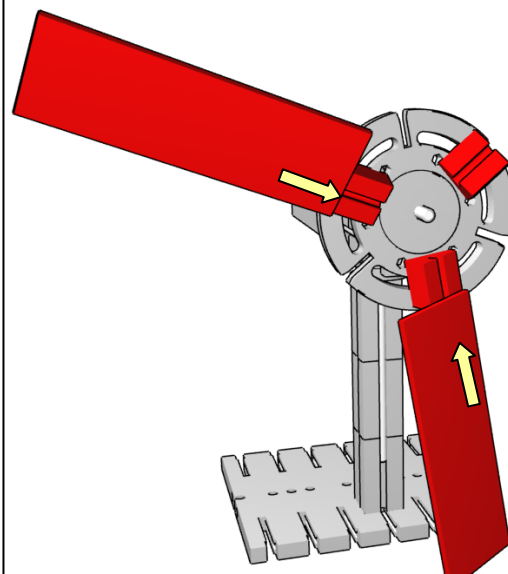
8. Flügelmontage
