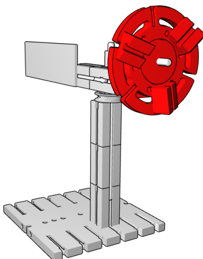
7. Einbau des Flügelrads
