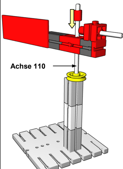
6. Einbau des Drehzapfens
