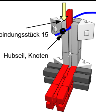
2. Kabinenboden
