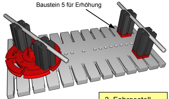
3. Fahrqestell
