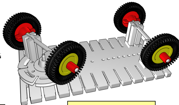
5. Radmontage
