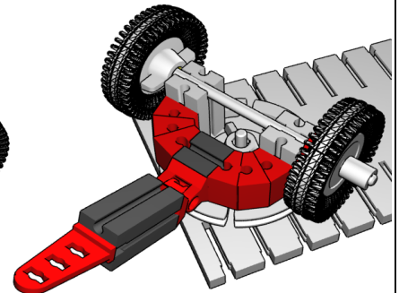
6. Anbau der Deichsel
