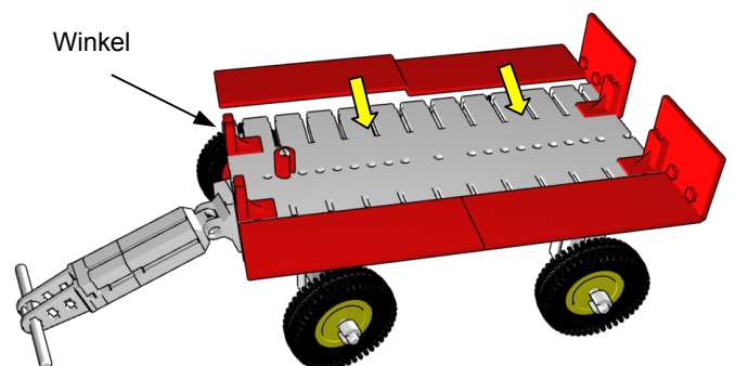
10. Anbau der Wände und Bodenplatten
