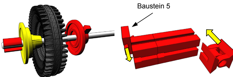
6. Räder mit Freilaufnaben
