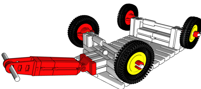
9. Anbau der Deichsel und der Räder
