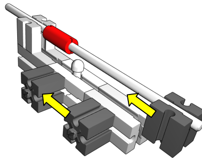
4. Einbau der Vorderachse
