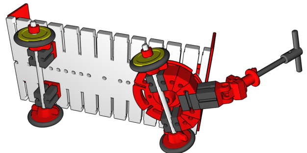
Modell 4b (vgl. Fahrgestelle 3.3.3.2 Bild 8a/b)
