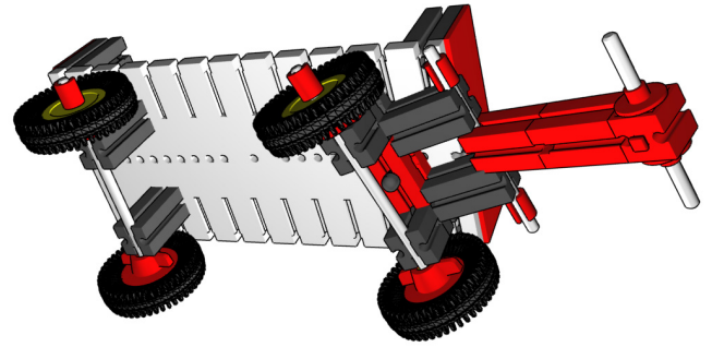
Modell 1b (Vgl. Wagenlenkungen 3.3.2.1 Bild 1a/b)
