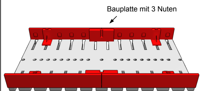
Bild 4 Niedrige Seitenwände
