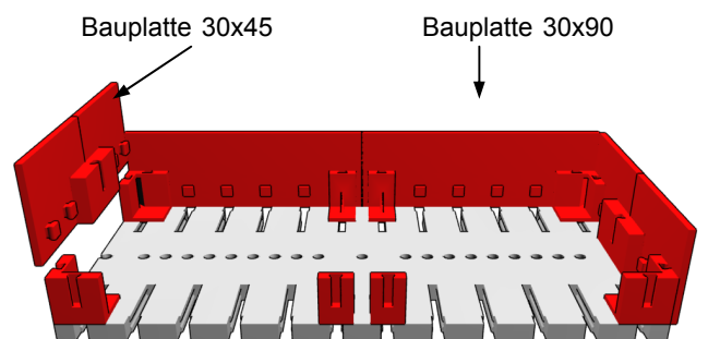
Bild 6 Geschlossener Kasten
