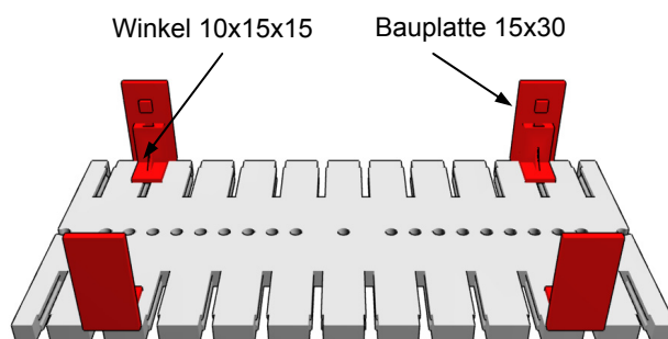
Bild 7 Halterungen für lange Teile
