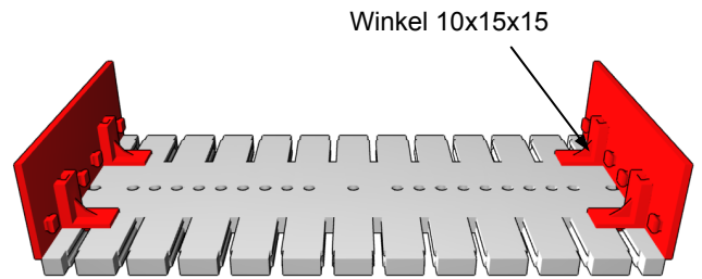
Bild 2 Aufbau mit Winkeln
