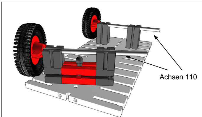
Bild 1a Fahrgestell mit Radabstand 60 mm
