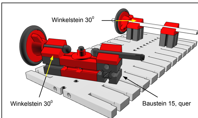
Bild 4a Fahrgestell mit kleinen Rädern
