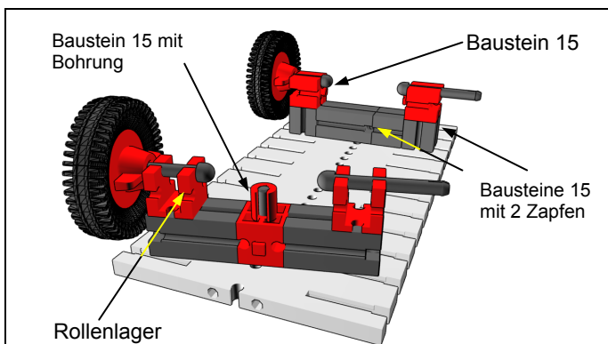
Bild 3a Fahrgestell mit Radabstand 75 mm
