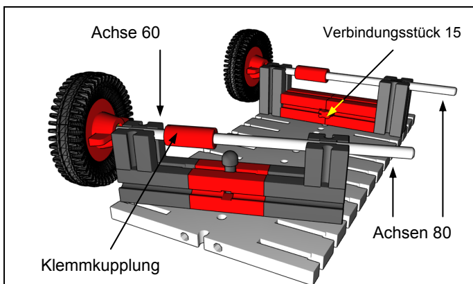
Bild 2a Fahrgestell mit Radabstand 90 mm
