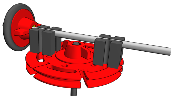
Bild 10a Drehschemel für kleine Räder
