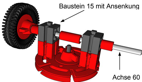
Bild 9a Drehschemel für großen Radabstand
