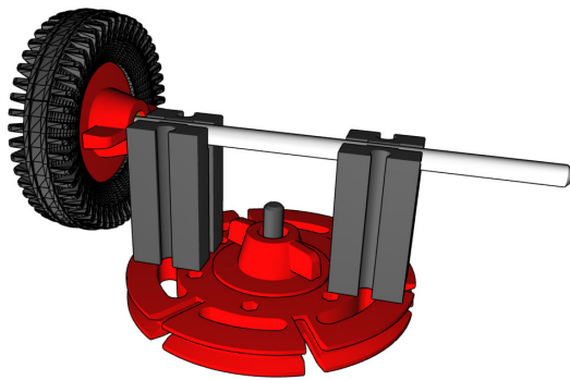
Bild 7a Drehschemel mit Drehscheibe
