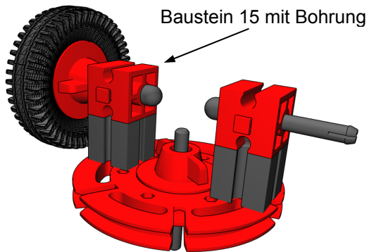
Bild 8a Drehschemel mit geteilten Achsen
