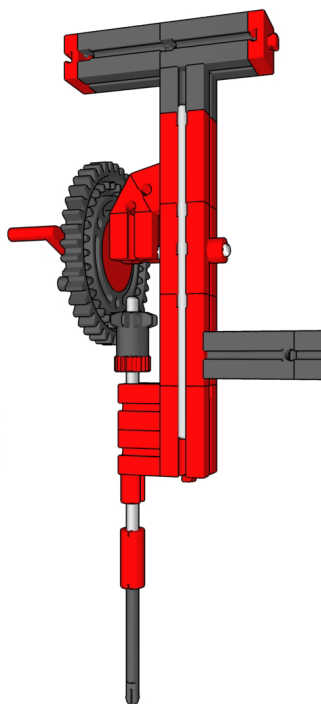
10.3.3 Übersetzung 1:3,2
