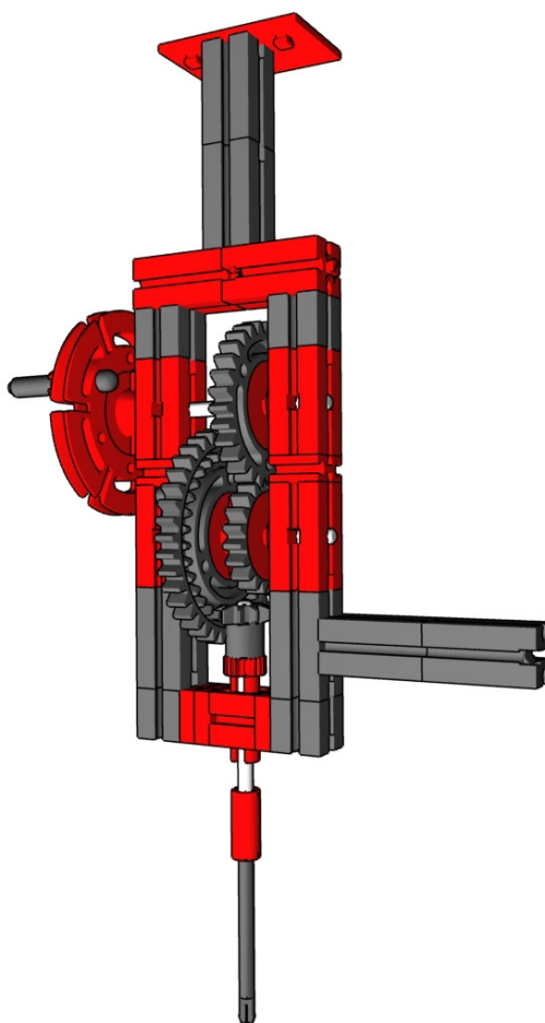
10.3.4 Übersetzung 1:4,8
