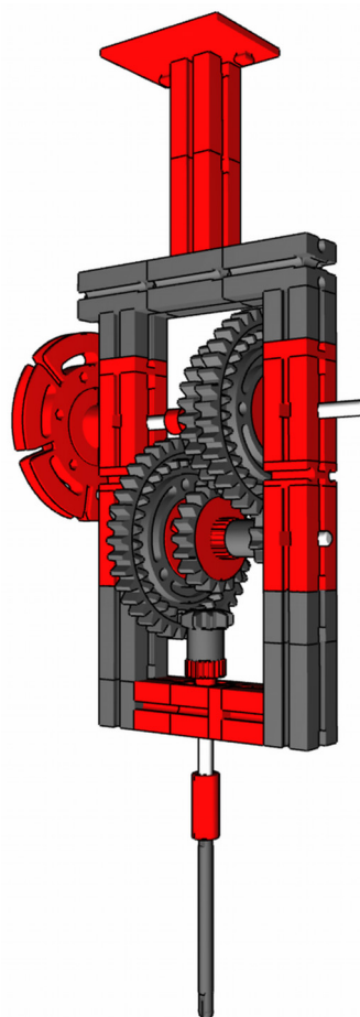
10.3.4 2 Übersetzungen 1:4,8 und 1:12,8
