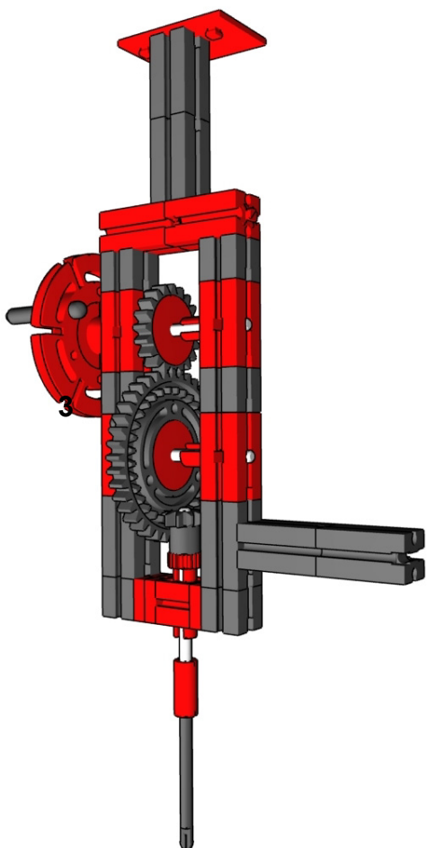
10.3.4 Übersetzung 1:1,6
