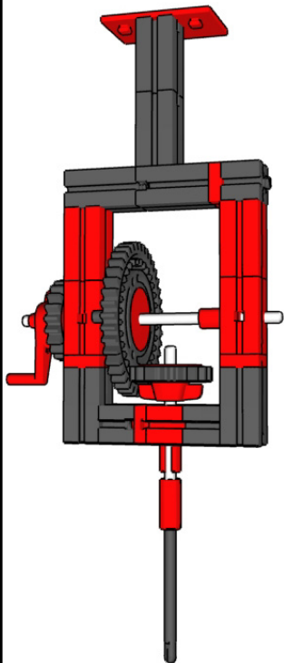
10.3.1 Übersetzung 1:1,6
