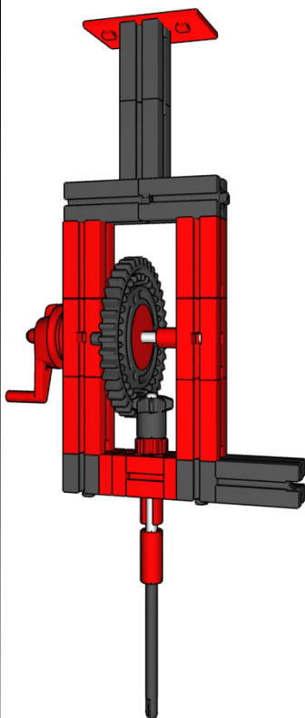
10.3.2 Übersetzung 1:3,2
