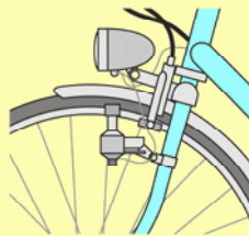
Reibrad- getriebe (kraft- schlüssig) z. B. beim Dynamo
