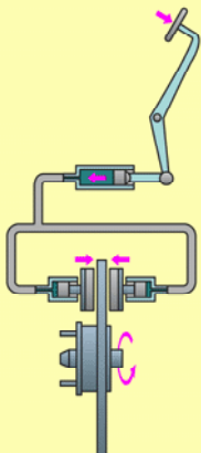
Druckmittel- getriebe z. B. hydrau- lisches Getriebe bei der Autobremse
